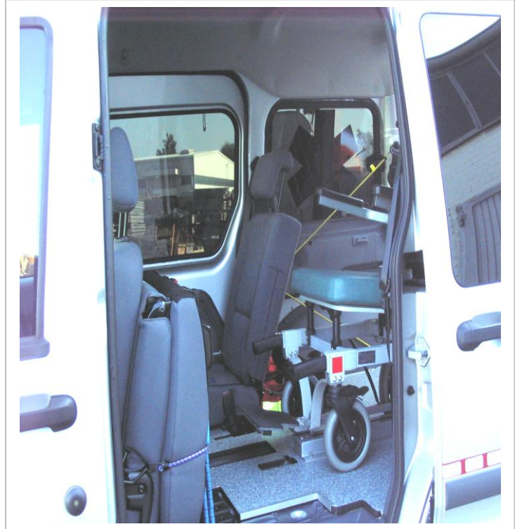
Ansicht über die Fahrzeugseitentür mit Tragestuhl
